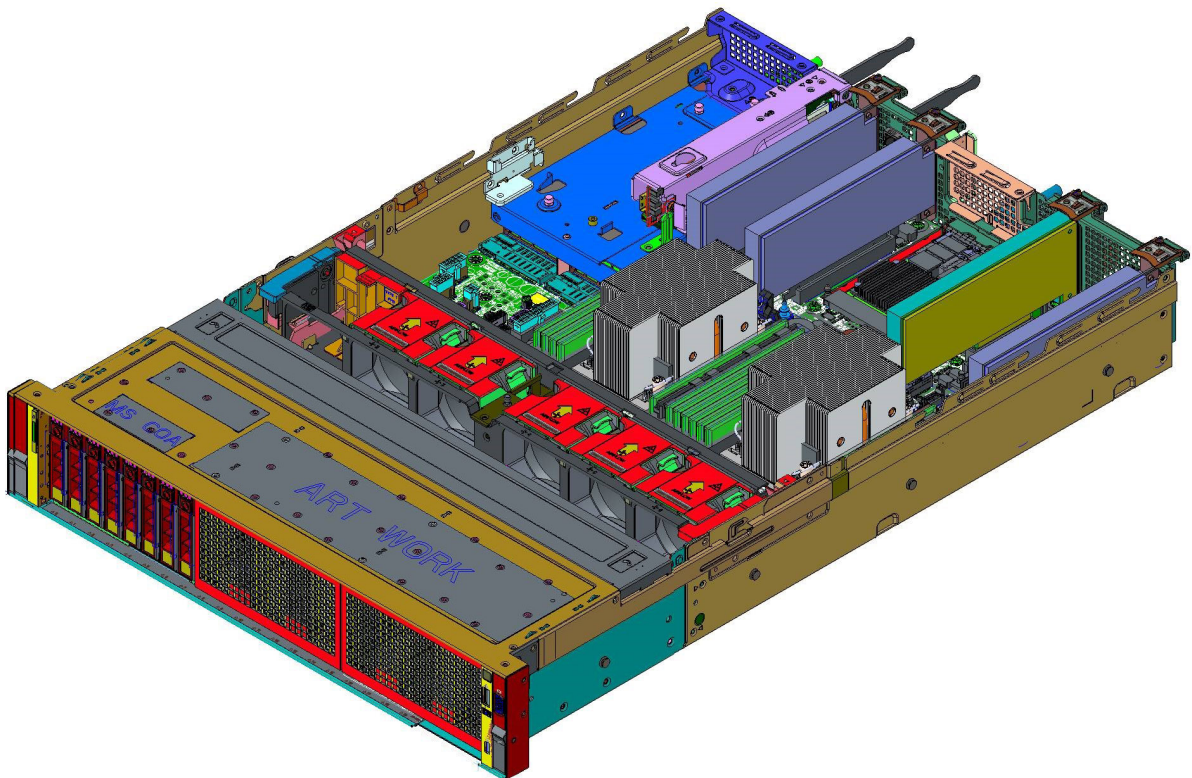
Ilustración 5. Interior del sistema de 8 unidades de 2,5 pulgadas
